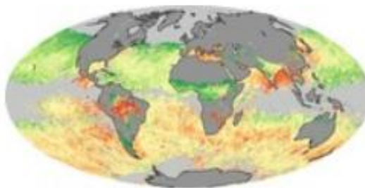
Aerosol Size
